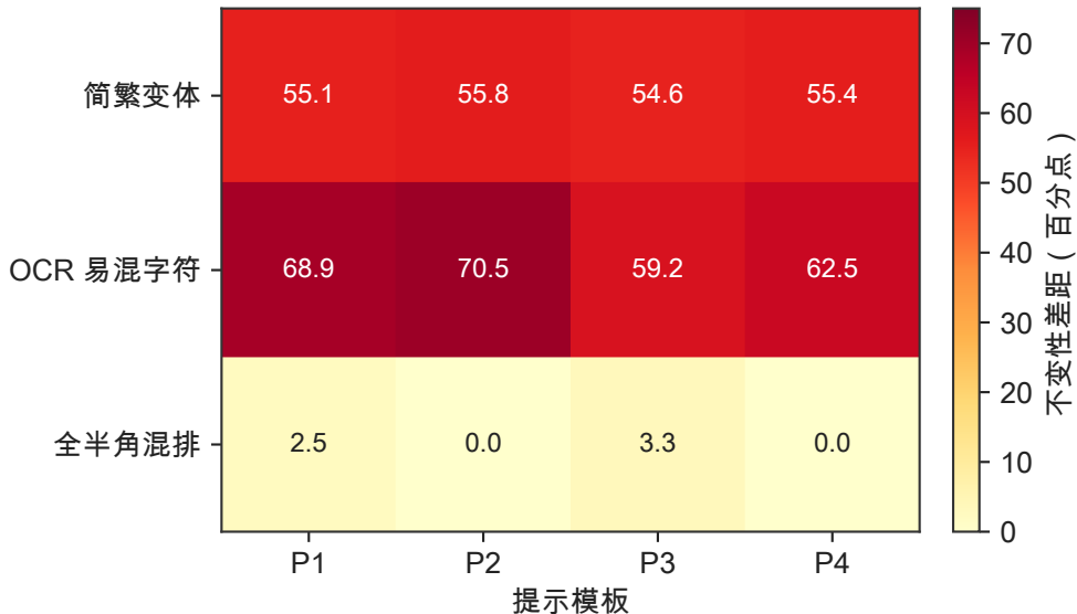
更强提示未消除规范不变性断裂
