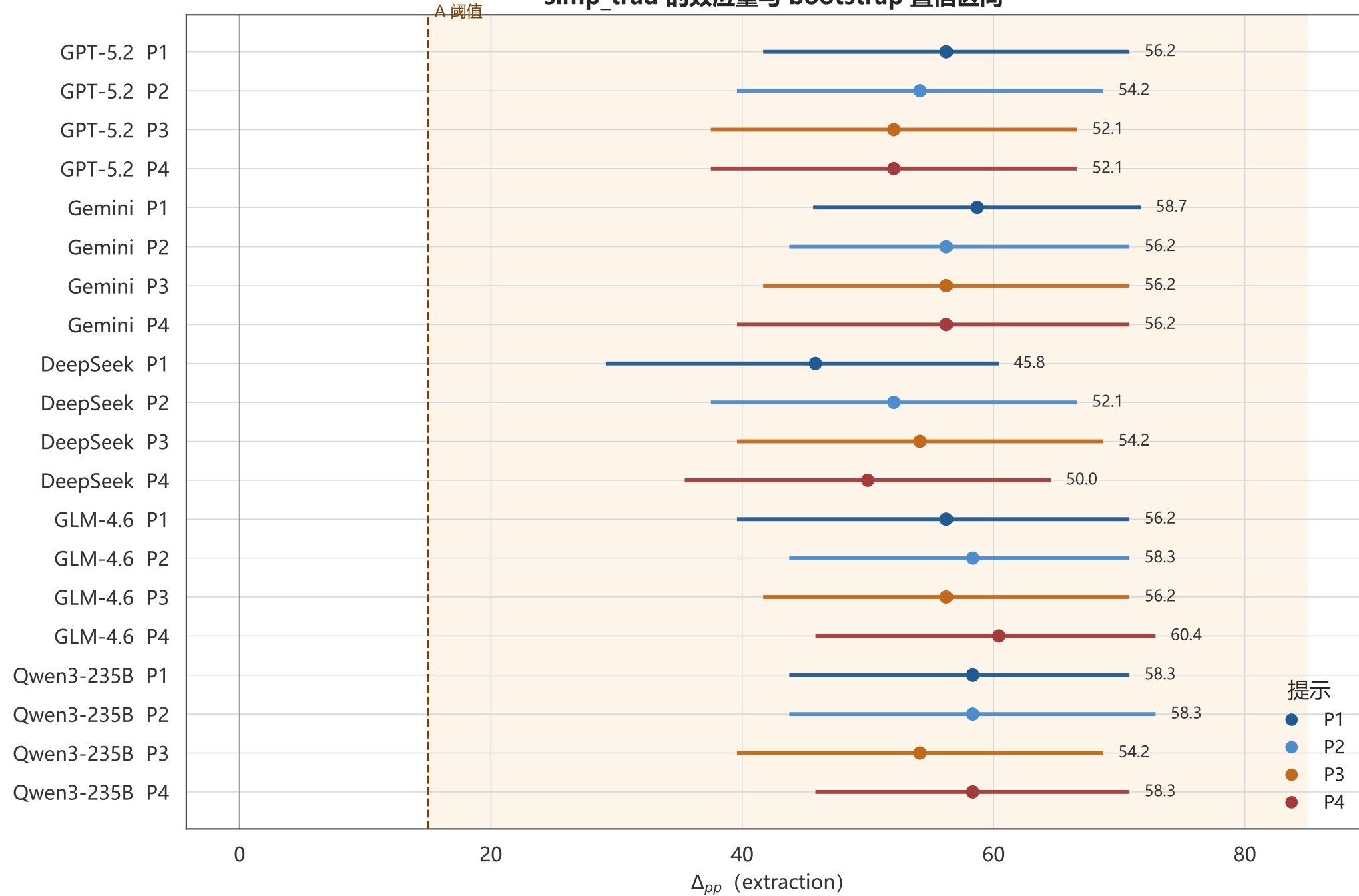
simp_trad 的效应量与 bootstrap 置信区间
