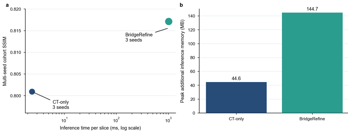
图 4: 统一 10 步、2 次递归协议下的独立效率测量。CT-only 与 BridgeRefine 在分进程中分别测量；时间不包含模型加载、输入传输和预处理，显存表示模型与输入分配后的额外推理峰值。
