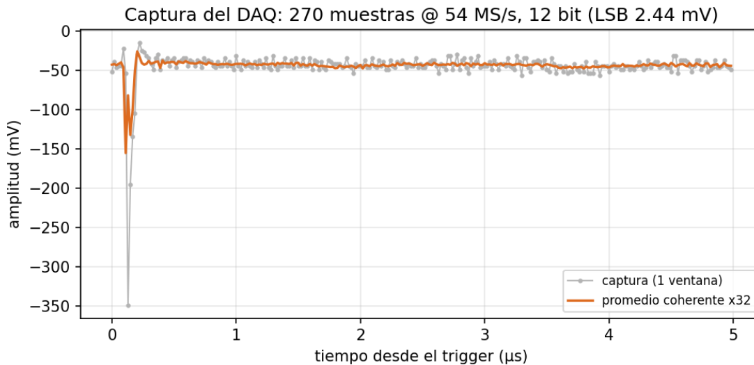
Figura 12: Captura del DAQ: ventana de 270 muestras @ 54 MSPS, 12 bit (LSB 2.44 mV); una adquisición individual y su promedio coherente \times 32 . Evidencia de captura a la velocidad y niveles especificados.
