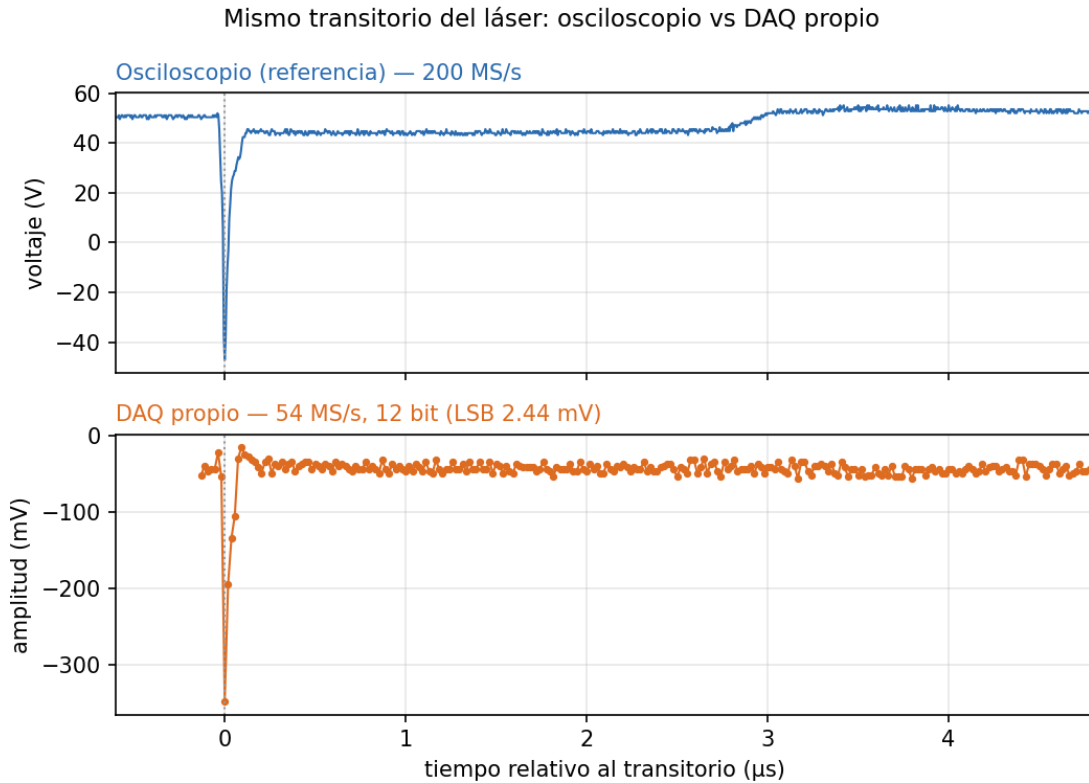
Figura 13: Mismo transitorio del láser capturado por el osciloscopio de referencia (200 MS/s) y por el DAQ propio (54 MS/s, 12 bit), alineados en el instante del evento. El DAQ reproduce el transitorio con timing coherente; las escalas verticales difieren por medir en puntos distintos del sistema.
