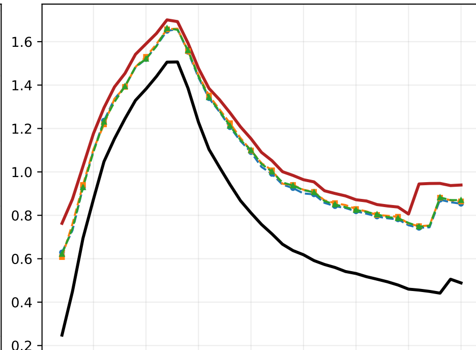
HST F555W - F814W vs. F814W
