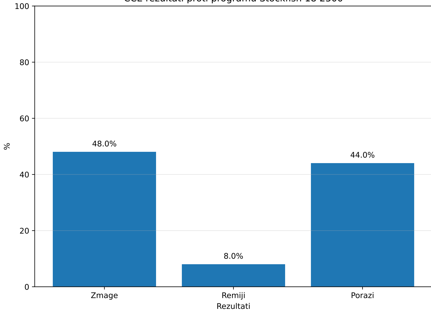
CCE rezultati proti programu Stockfish 18 2300
