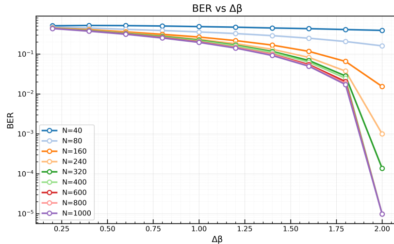
Slika 6.2: BER v odvisnosti od razlike \Delta\beta pri različnih vrednostih N .
