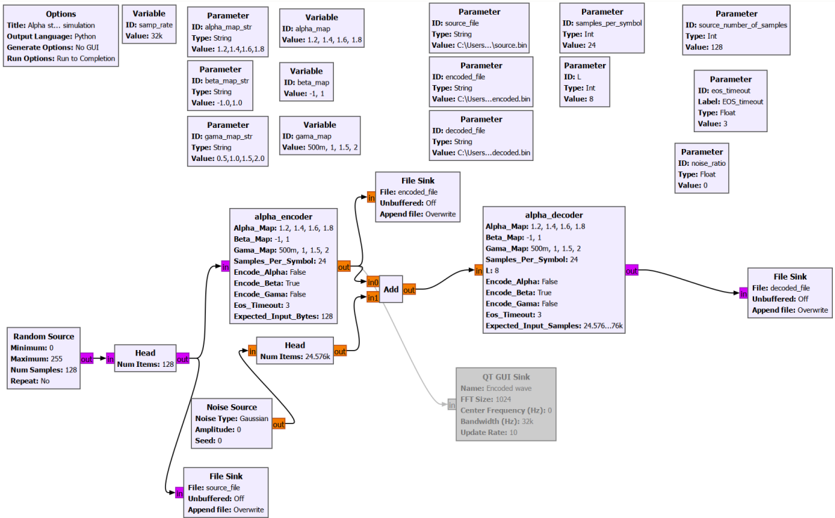
Slika 5.1: Blokovni diagram komunikacijskega sistema v GNU Radio Companion.
