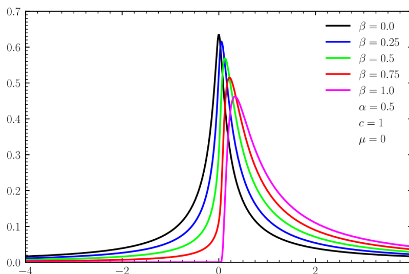
Slika 3.2: Graf za različne parametre \beta [? ].
