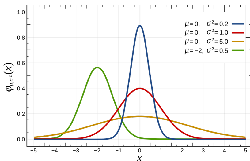
Slika 3.3: Gostote verjetnosti normalnih porazdelitev za različne vrednosti parametrov [? ].
