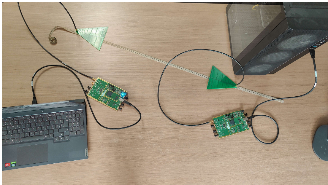
Slika 6.4: Eksperimentalni komunikacijski sistem z napravama USRP B210, log-periodičnima antenama WA5VJB LP8565A2 ter računalnikoma oddajnika in sprejemnika.
