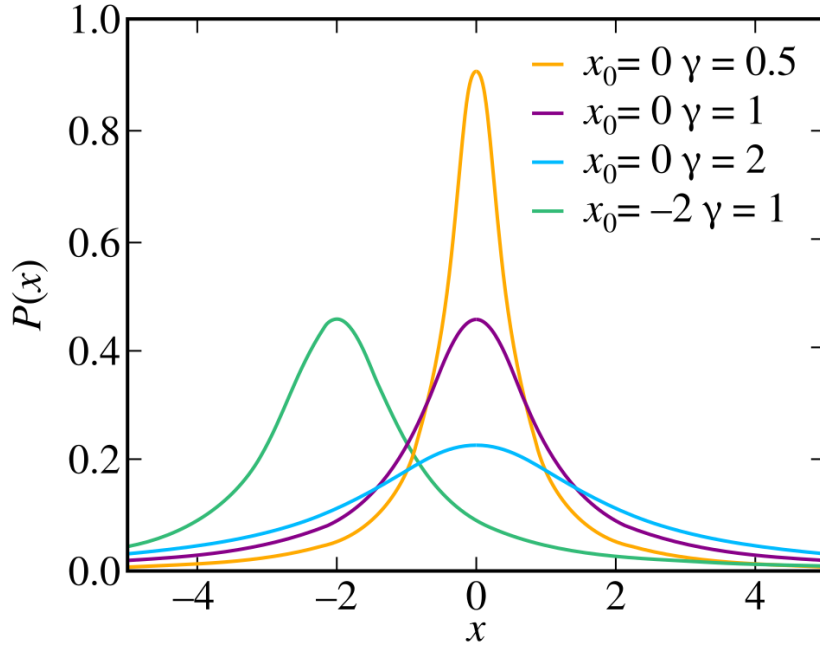
Slika 3.4: Gostote verjetnosti Cauchyjevih porazdelitev za različne vrednosti parametrov [? ].
