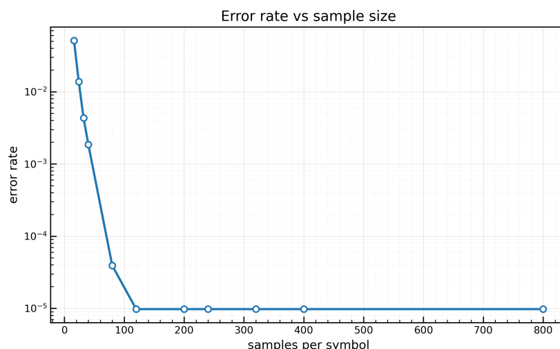
Slika 5.4: Graf BER glede na velikost vzorca
