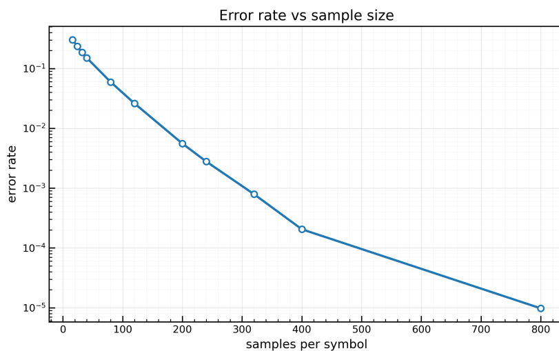
Slika 5.5: Graf BER glede na velikost vzorca s šumom
