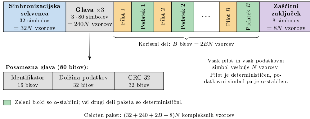
Slika 5.2: Struktura posameznega oddajnega paketa pri komunikaciji prek opreme SDR. Sinhronizacijski sekvenci in trikrat ponovljeni glavi sledijo pari pilotskih in \alpha -stabilnih podatkovnih simbolov ter zaščitni zaključek.
