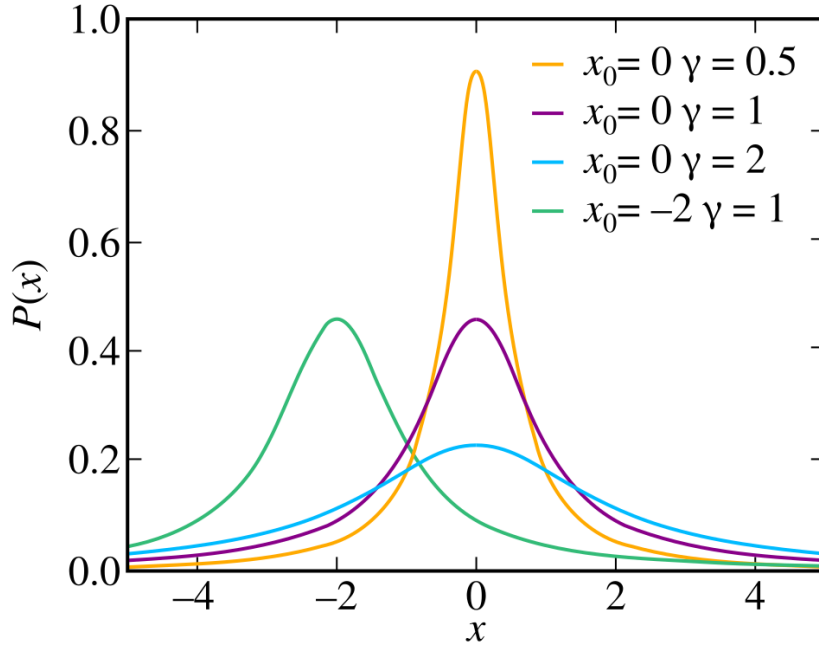
Slika 3.4: Gostote verjetnosti Cauchyjevih porazdelitev za različne vrednosti parametrov [19].
