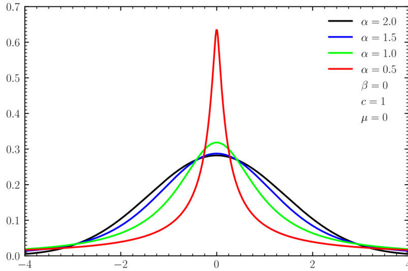
Slika 3.1: Graf za različne parametre \alpha [22].
