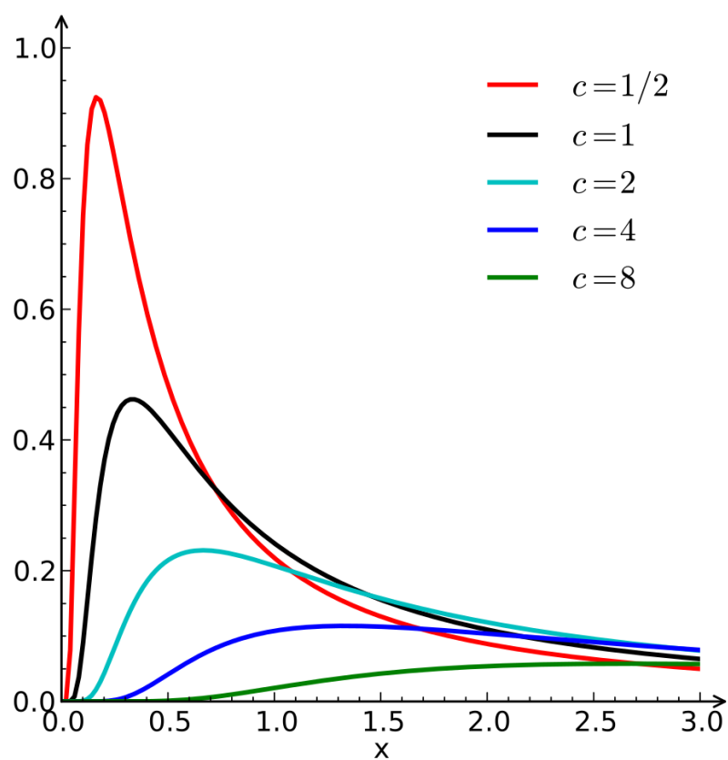
Slika 3.5: Gostote verjetnosti Lévyjevih porazdelitev za različne vrednosti parametrov [20].
