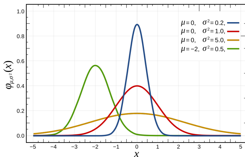
Slika 3.3: Gostote verjetnosti normalnih porazdelitev za različne vrednosti parametrov [21].
