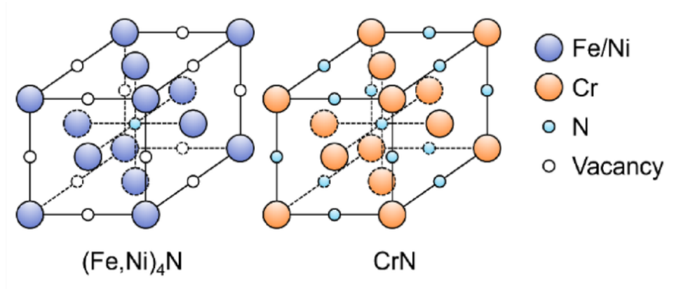
Figure 16. Fe/Ni 질화물과 CrN 결정구조 비교. 출처: Jeong and Yeom [1], Fig. 14, CC BY-NC-ND 4.0.
