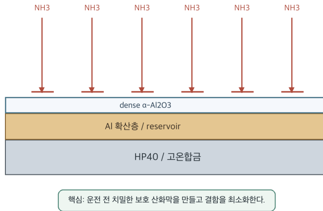
Figure 7. 알루미나 형성 확산코팅을 이용한 고압 암모니아 크래킹용 합금 보호 개념.
