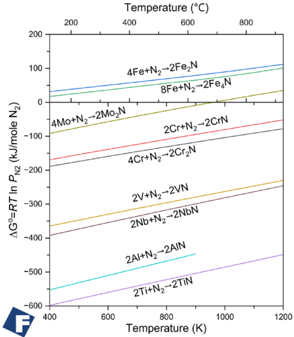
Figure 13. 대표 금속 질화물 형성 반응의 Gibbs 자유에너지 비교. 출처: Jeong and Yeom [1], Fig. 4, CC BY-NC-ND 4.0.
