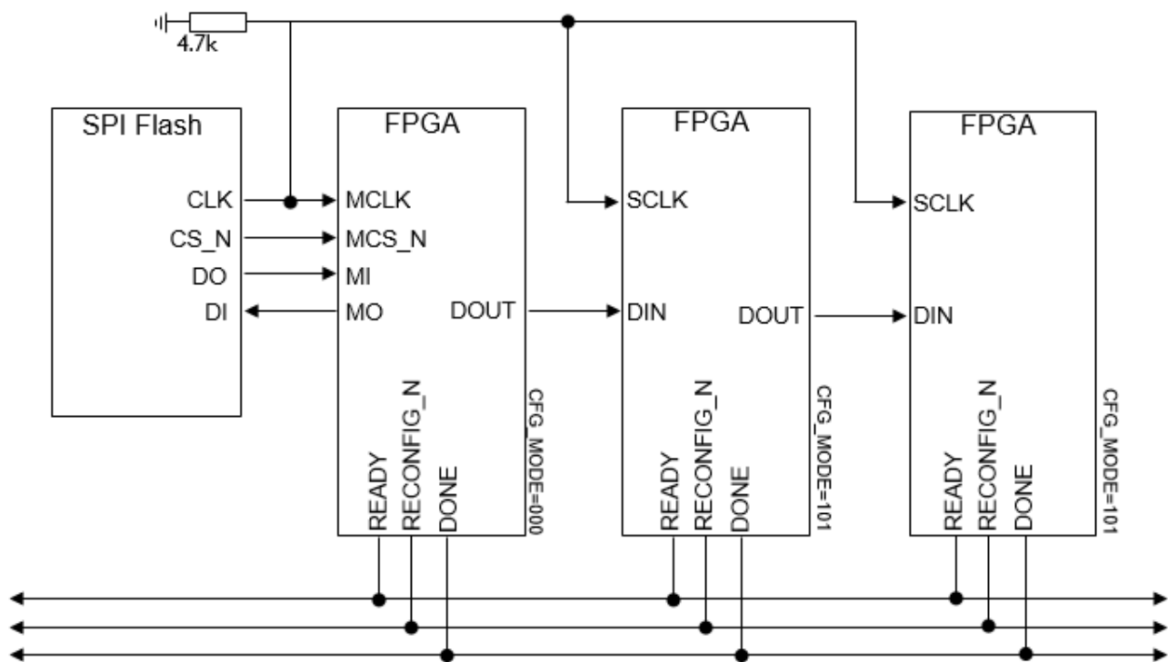
图 7-55 一片 Flash 配置多片 FPGA 连接示意图
