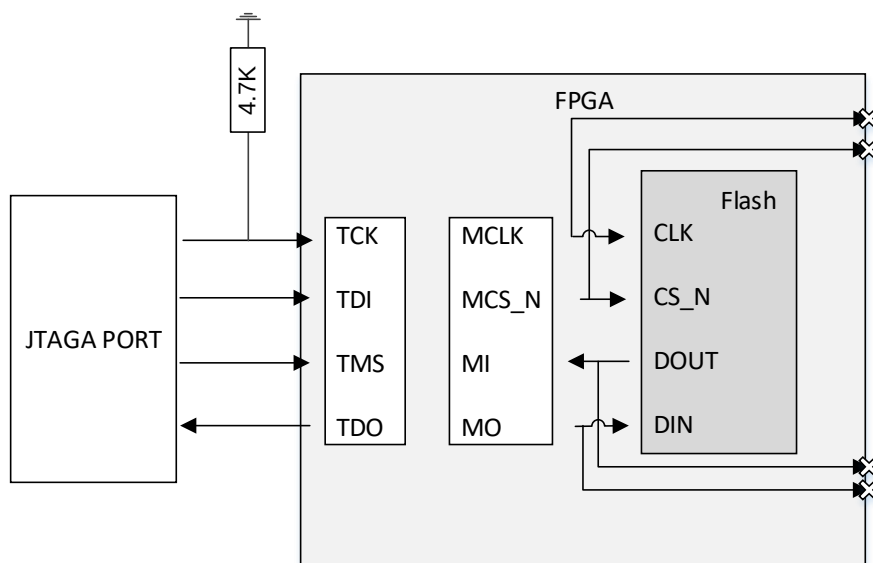
图 7-27 JTAG 接口编程内嵌 SPI-Flash 连接示意图（GW2ANR-18/GW2AN-55/GW1AN-1/GW1AN-1S）
