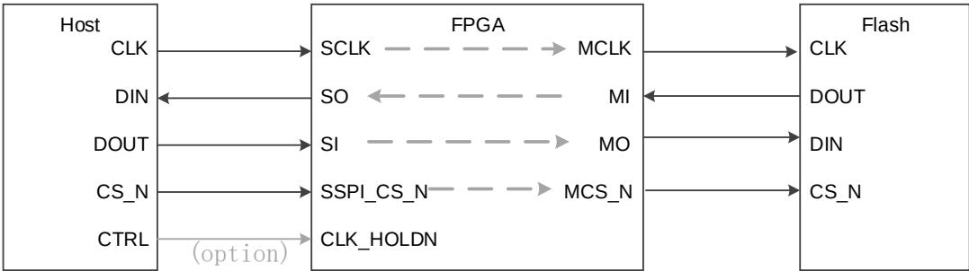
图 7-42 SSPI 编程外部 Flash 连接示意图(GW2A-18/55,GW1N(R)-9, GW1NS-4/4C)
