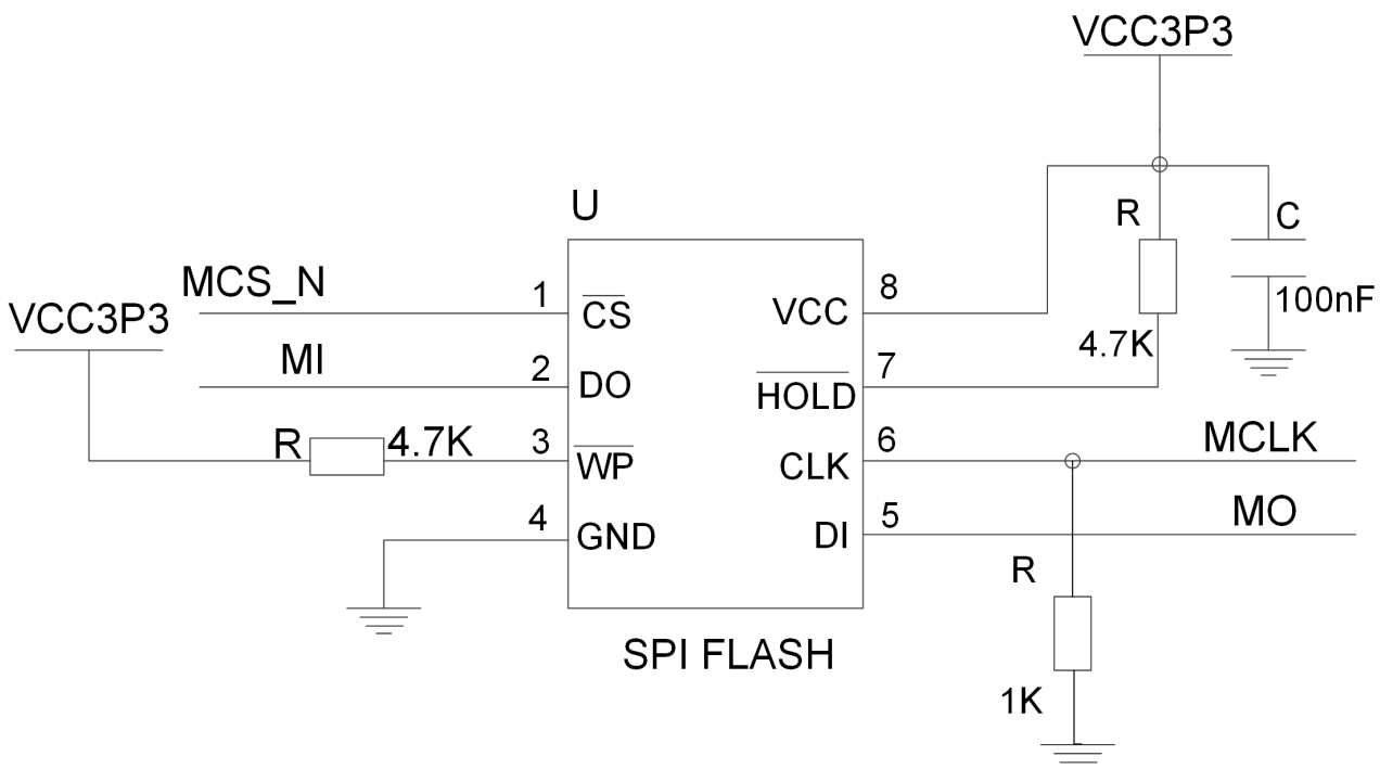
图 4 MSPI 电路
