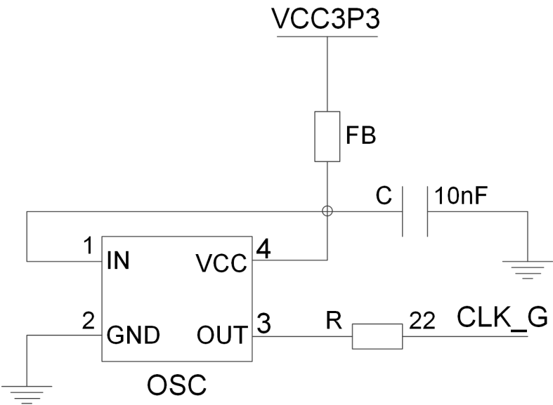
图 7 FPGA 外接晶振电路
