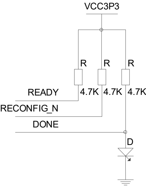
图 5 READY、RECONFIG_N、DONE 参考电路
