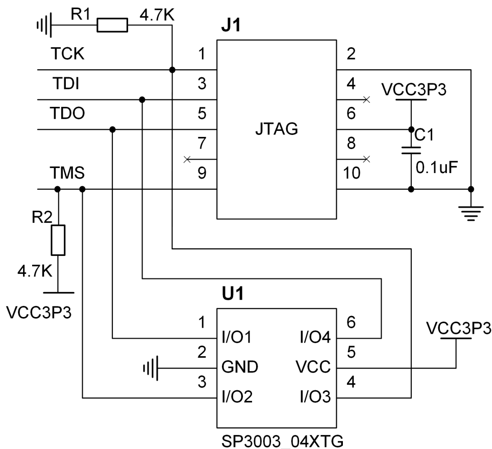
图 3 JTAG 电路
