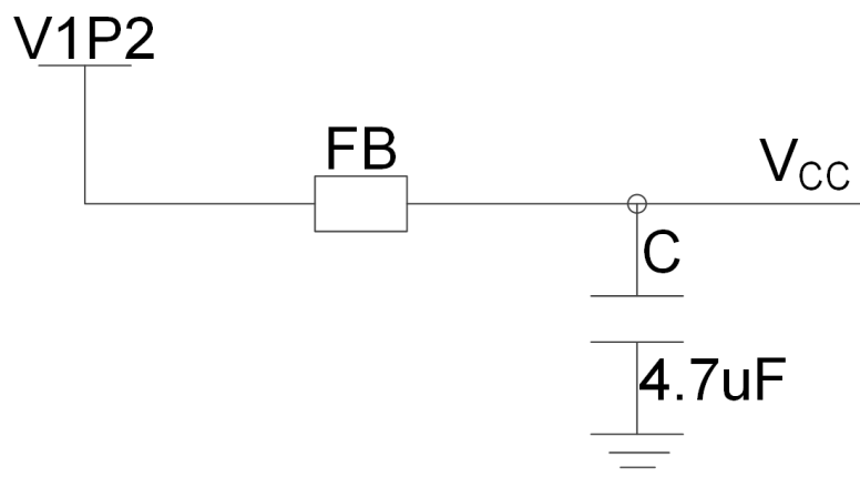
图 2 V_{CC} 核电压输入端噪声处理
