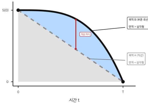
Figure 4: 꺾적 A(직선) 와 꺾적 B(위로 부푼 곡선) 의 적분값 비교
