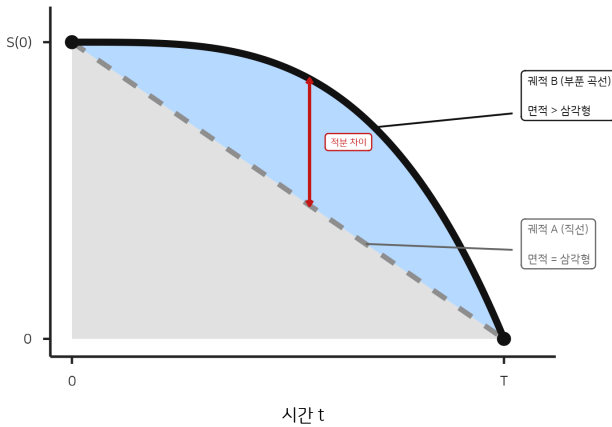
Figure 4: 궤적 A(직선) 와 궤적 B(위로 부분 곡선) 의 적분값 비교
