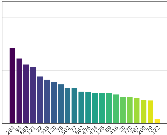
ICVul
