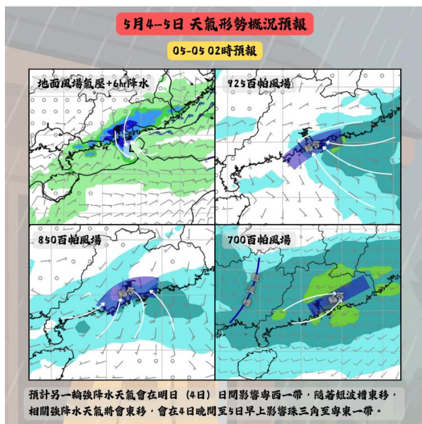
（05-04—05 天氣形勢概況預報圖）
