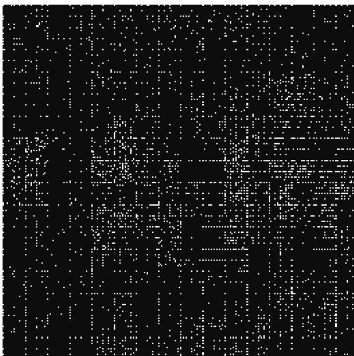
QFT
