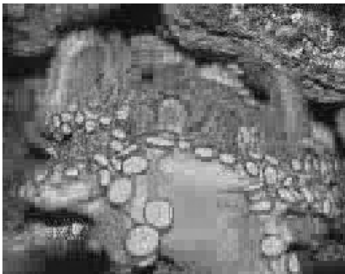
QFT
