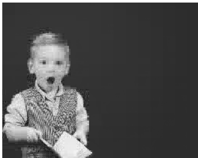
QFT
