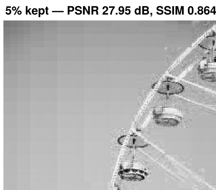
QFT
