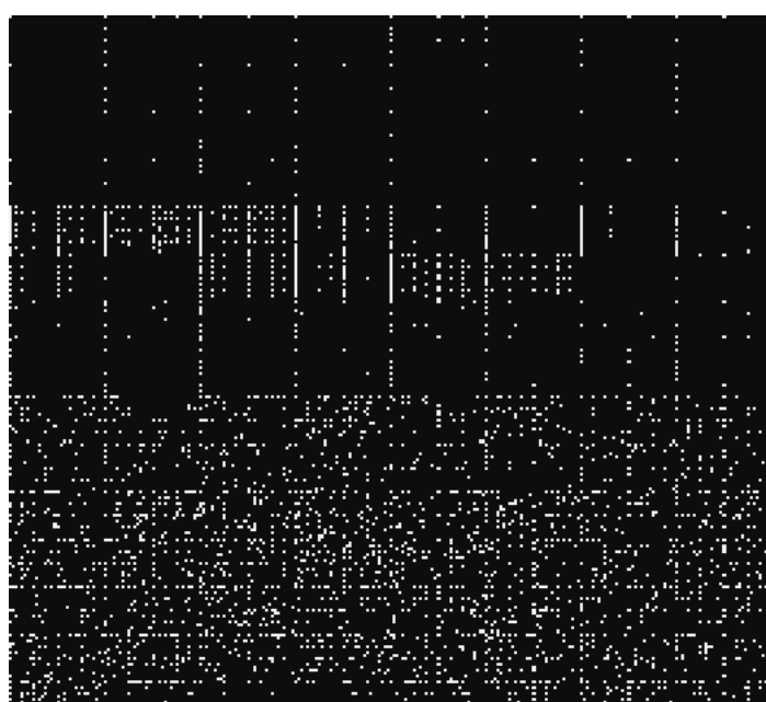
QFT
