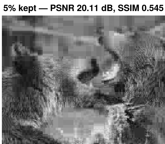
QFT
