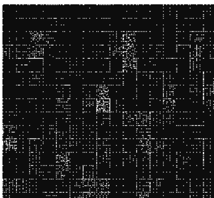
QFT
