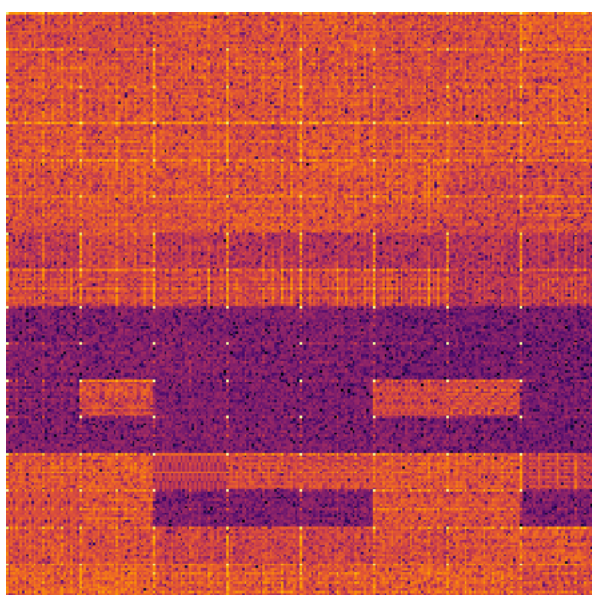
TEBD
