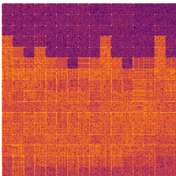
QFT
