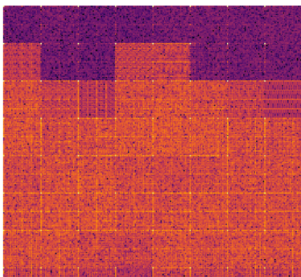
MERA
