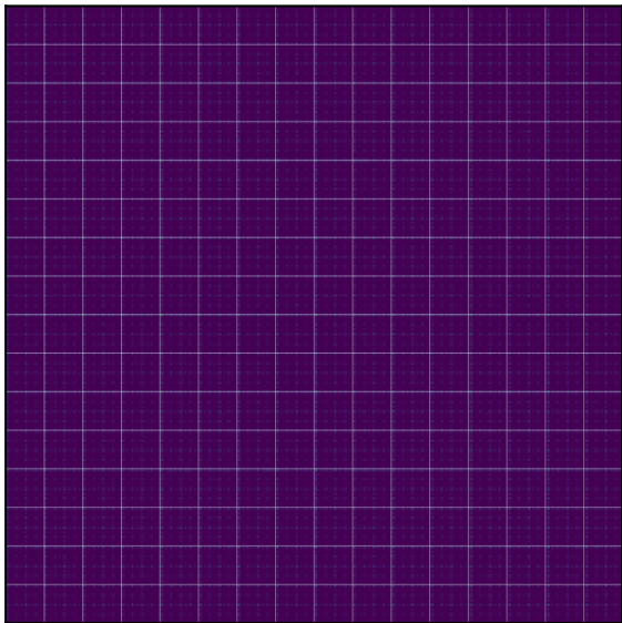
untrained global QFT
