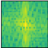
fft
