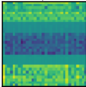
qft
