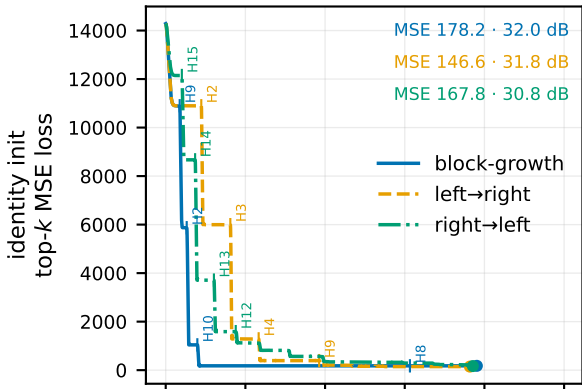
DIV2K (m=n=8)
