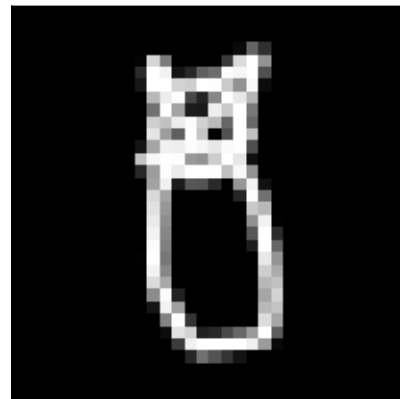
PSNR 91.86 dB
