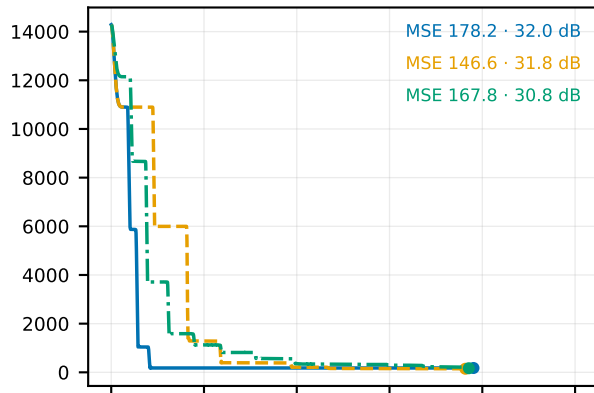
DIV2K (m=n=8)
