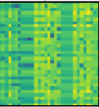
qft
