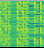
tebd
