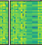
entangled_qft
