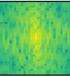
fft
