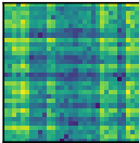
DCT-IV
