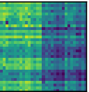
TEBD
