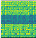
QFT
