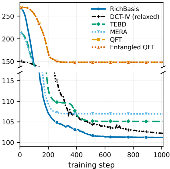
validation MSE
