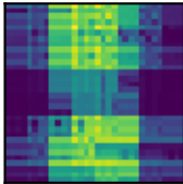
tebd
