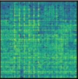
TEBD
