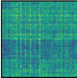
DCT-IV
