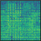
TEBD
