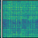
DCT-IV
