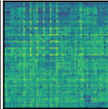
MERA
