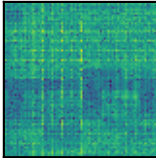
QFT
