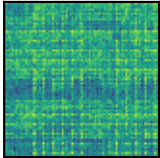
RichBasis
