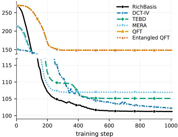
validation MSE
