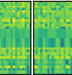
entangled_qft
