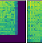
bd_pca
