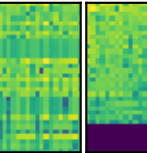
tebd
