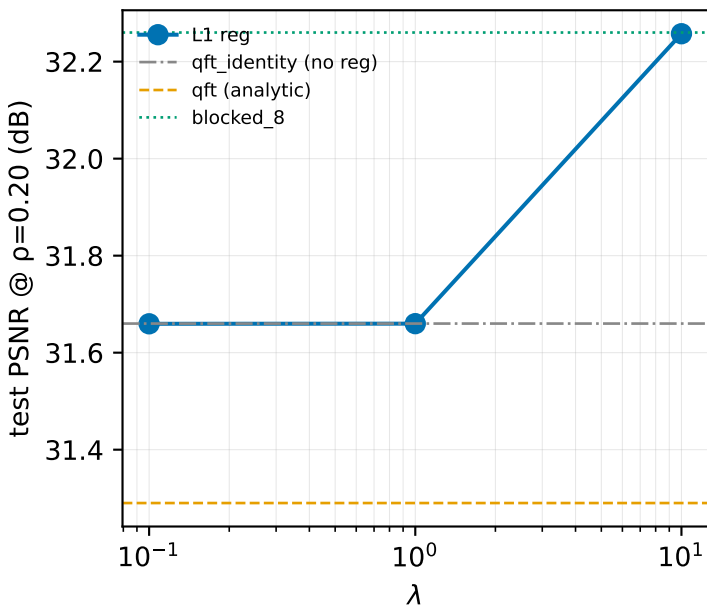
DIV2K-8q (m=n=8)
