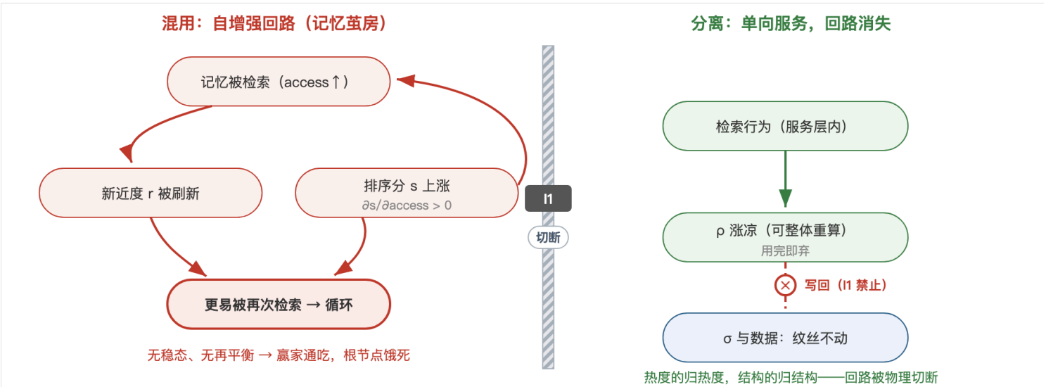
左：混用形态下，检索刷新新近度（Generative Agents 的 0.995 衰减按最近访问计）， \partial s / \partial \text{access} > 0 构成自增强回路，无稳态与再平衡机制时终局为赢家通吃。右：I1 将访问敏感性关进服务层并禁止写回持久字段，回路被物理切断；对照人脑：测试效应的强化有突触稳态与睡眠巩固再平衡配平——“要学就学全”。
