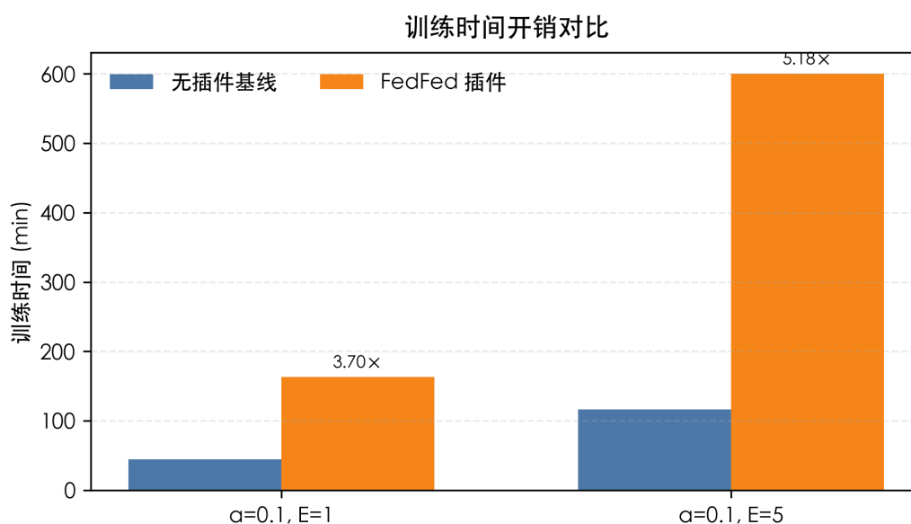
图 5-14 FedFed 插件训练时间开销对比
