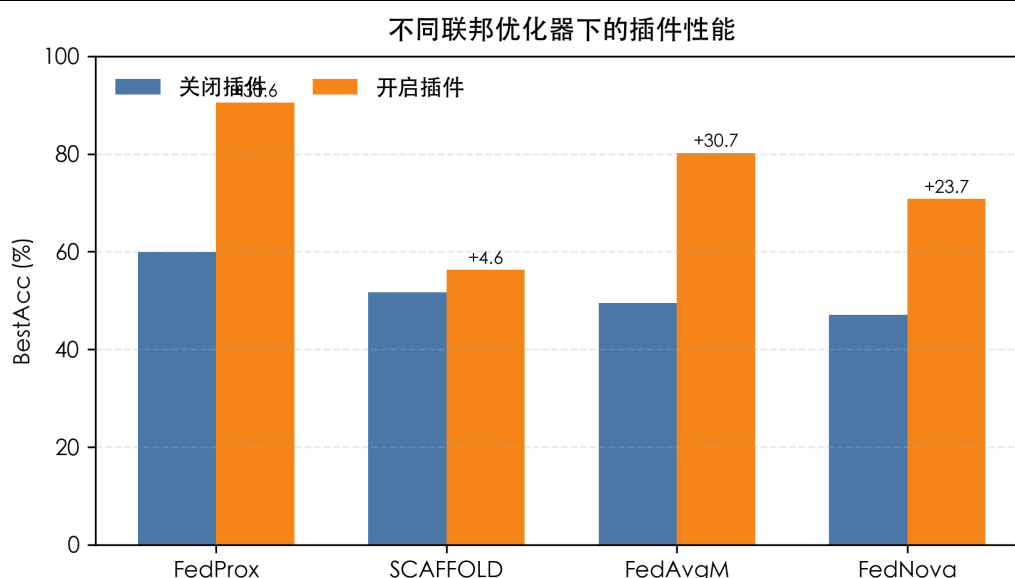
图 5-13 不同联邦优化器下的插件性能对比
