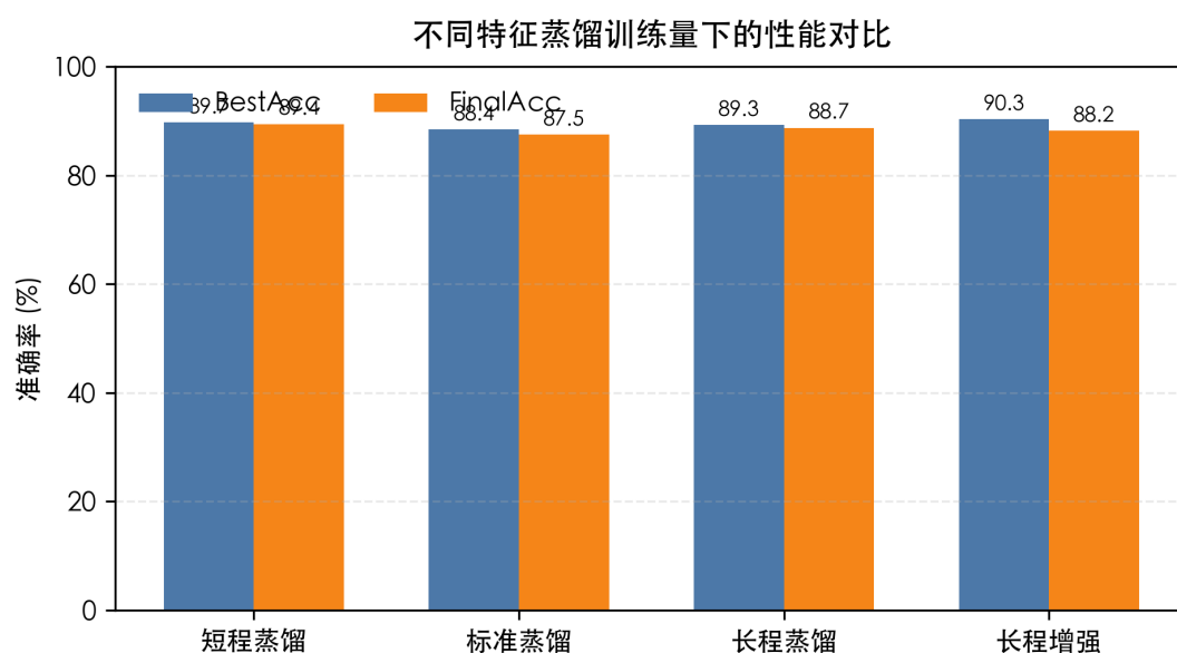
图 5-7 不同特征蒸馏训练量下的性能对比
