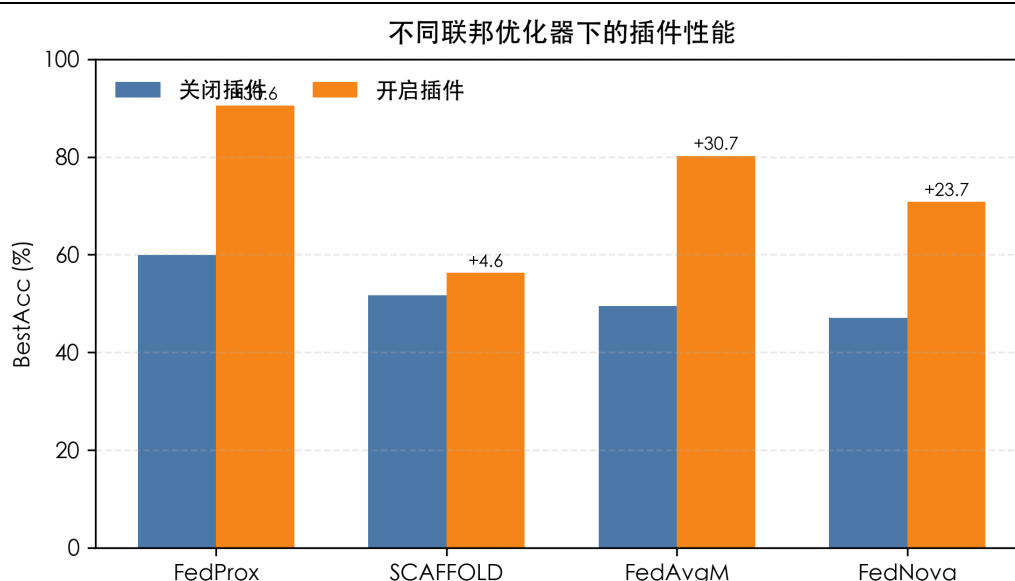
图 6-6 不同联邦优化器下的插件性能对比
