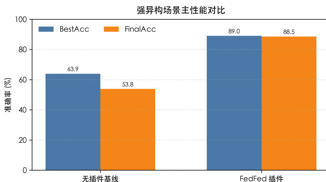
图 5-1 强异构场景下主性能对比
