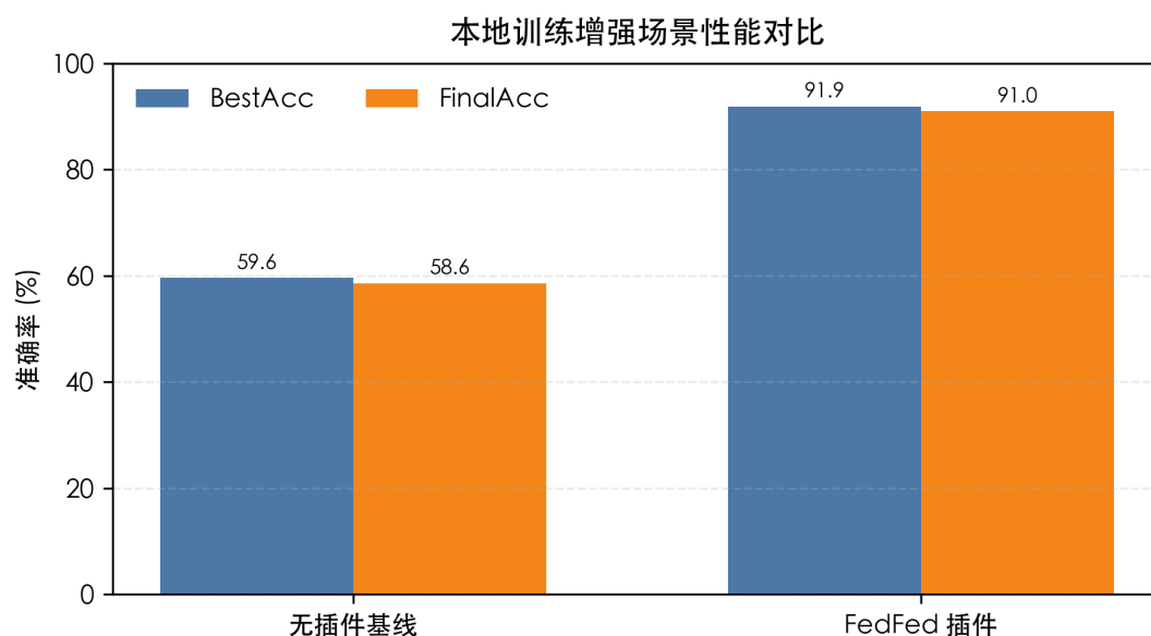
图 5-5 本地训练强度增大时的性能对比
