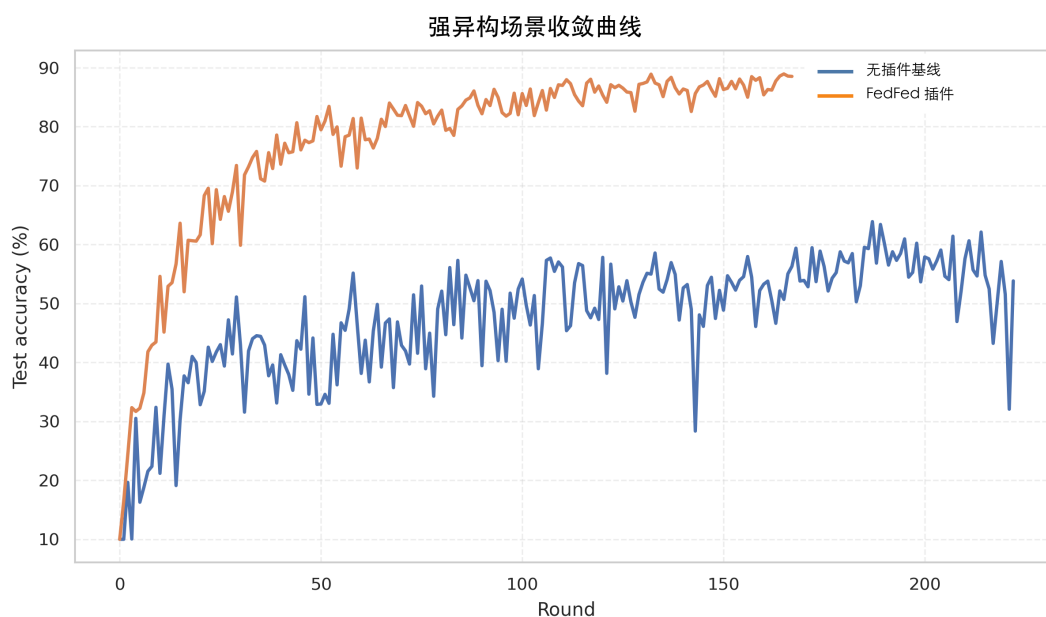
图 5-2 强异构场景下的收敛曲线
