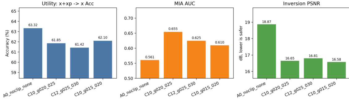
图 6-5 不同配置下的性能与隐私指标对比
