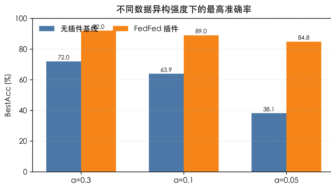
图 5-3 不同数据异构强度下的性能对比
