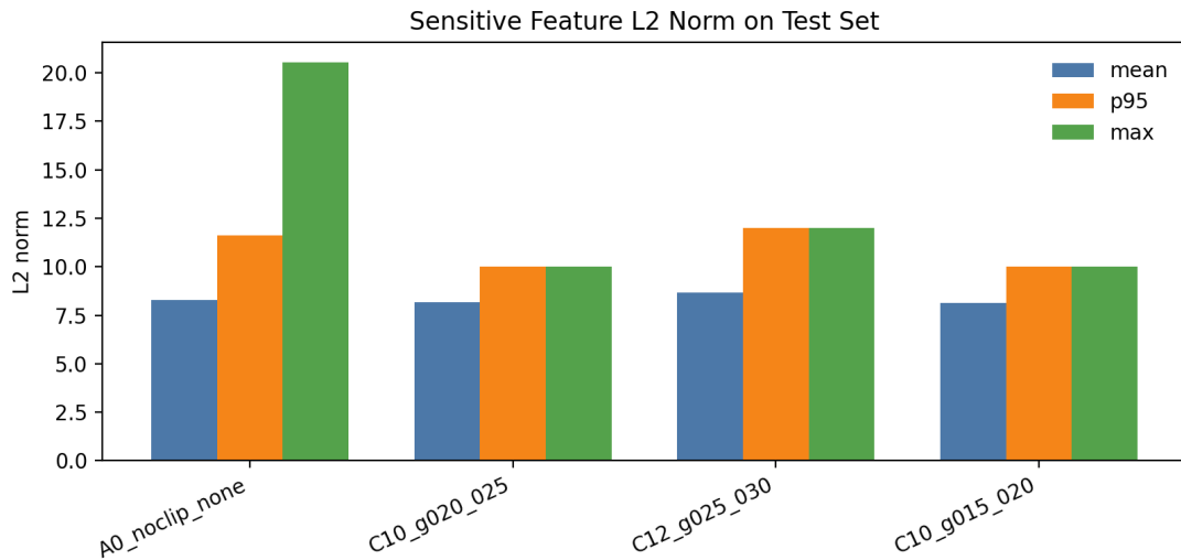
图 6-2 敏感特征 L2 范数统计对比
