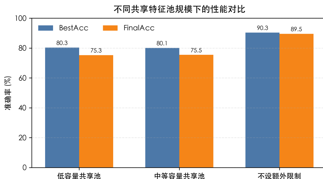
图 5-6 不同共享特征池规模下的性能对比
