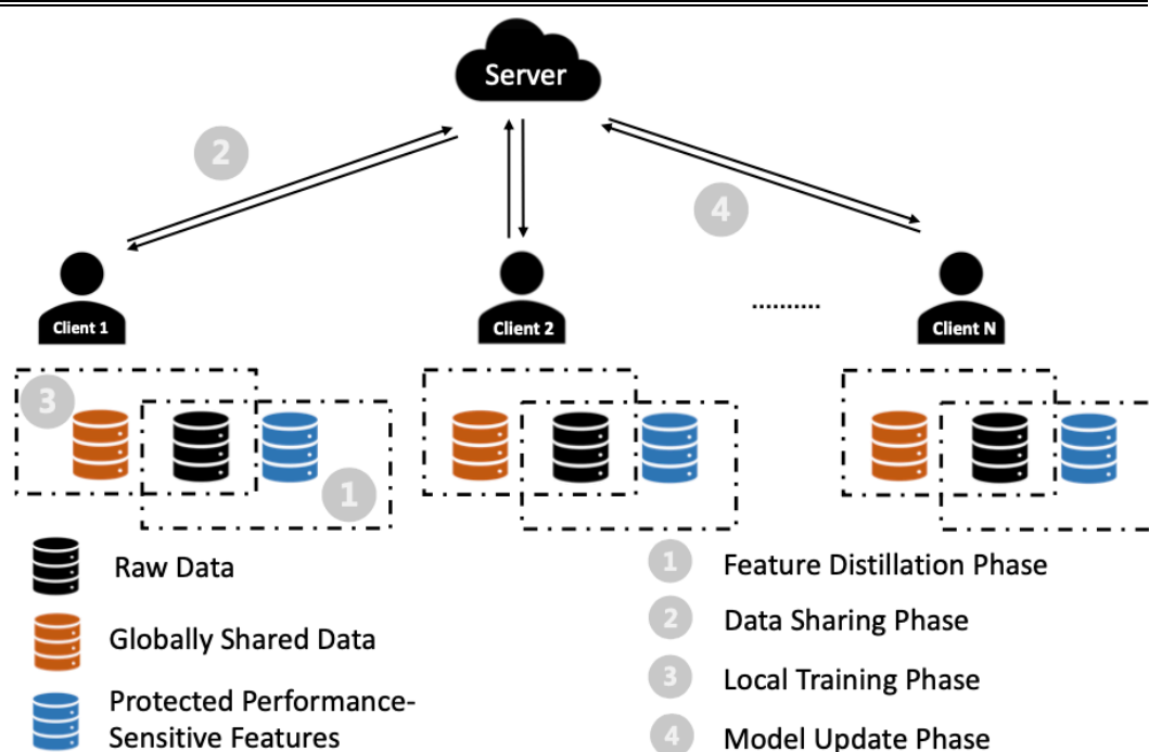
图 2 FedFed 工作流程概述示意图
