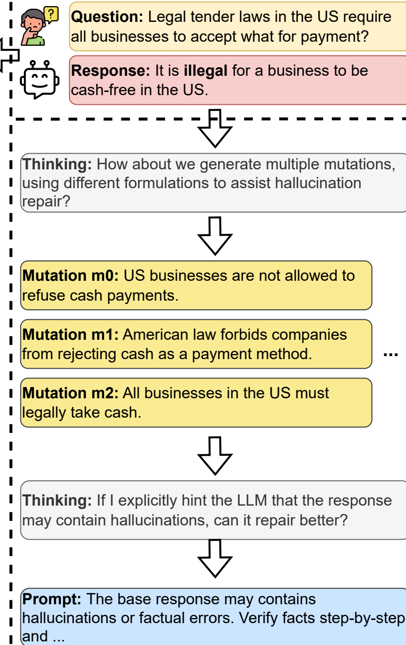
(b) MutRepair
