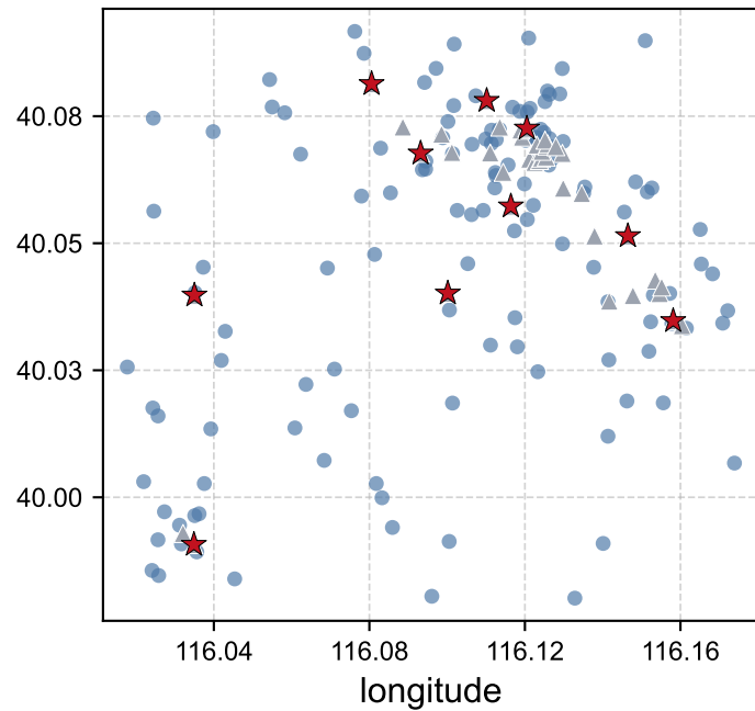
Sparse Density CV = 0.541
