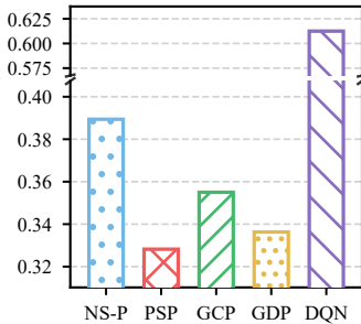
(b) # users (130).
