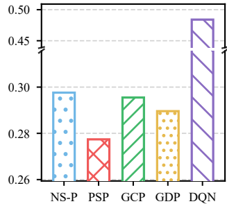
(d) # users (180).
