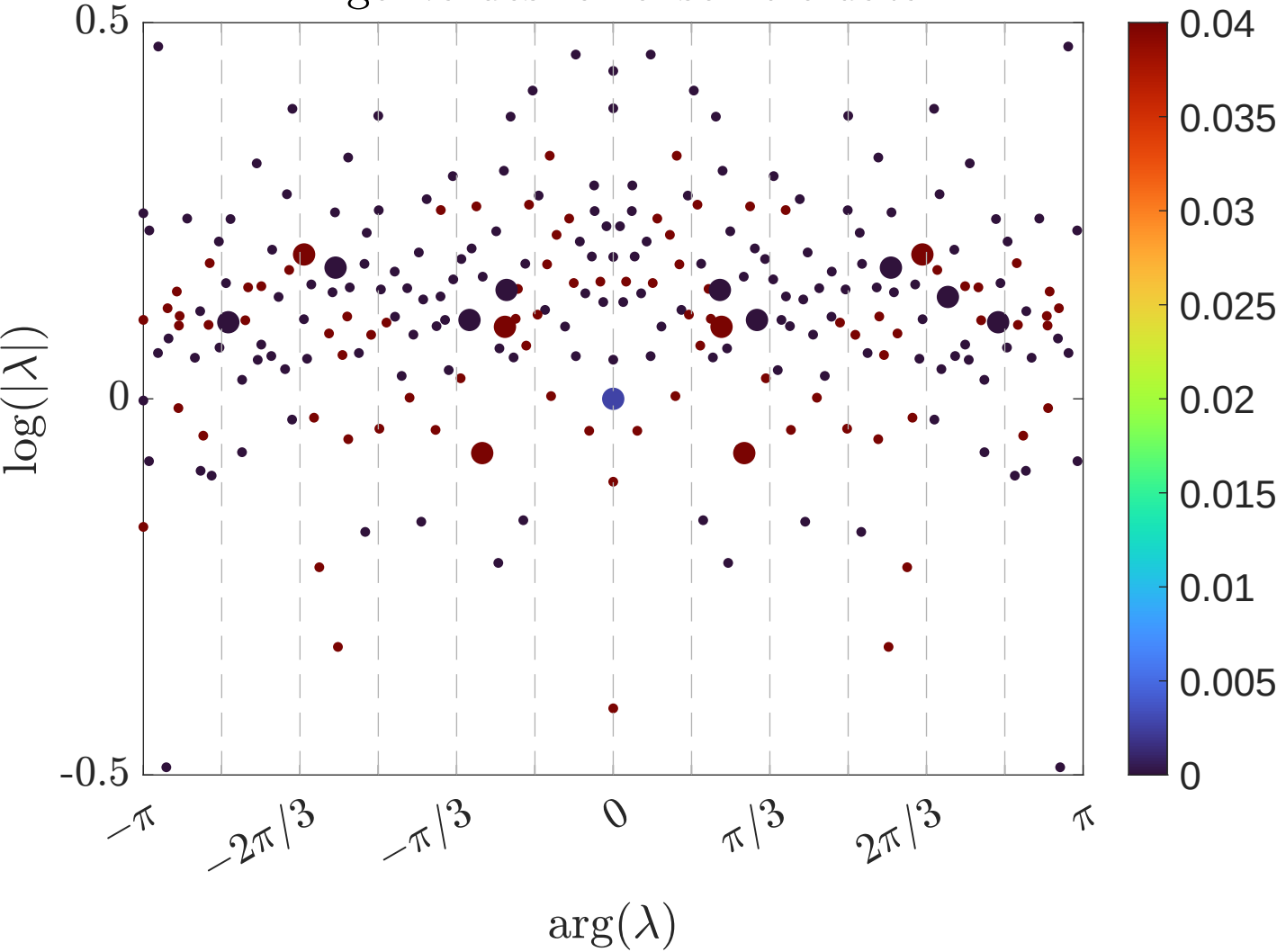
Eigenvalues for ensemble data
