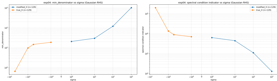
图 16: Modified vs True Helmholtz: 频域分母最小值 d_{\min} (左) 与谱条件数指标 (右)
