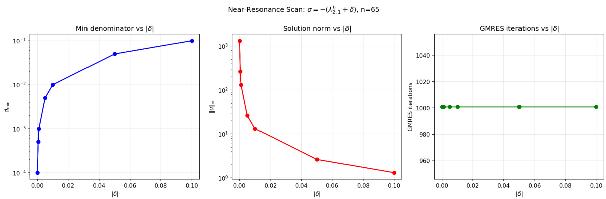
图 18: 近共振扫描： d_{\min} 、解范数和 GMRES 迭代次数随 |\delta| 变化（ n = 65 ，目标模态 (2, 1) ）
