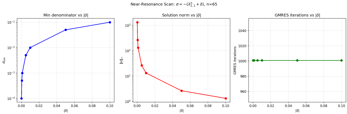
图 6: True Helmholtz 近共振扫描: d_{\min} 、解范数和 GMRES 迭代随 |\delta| 的变化
