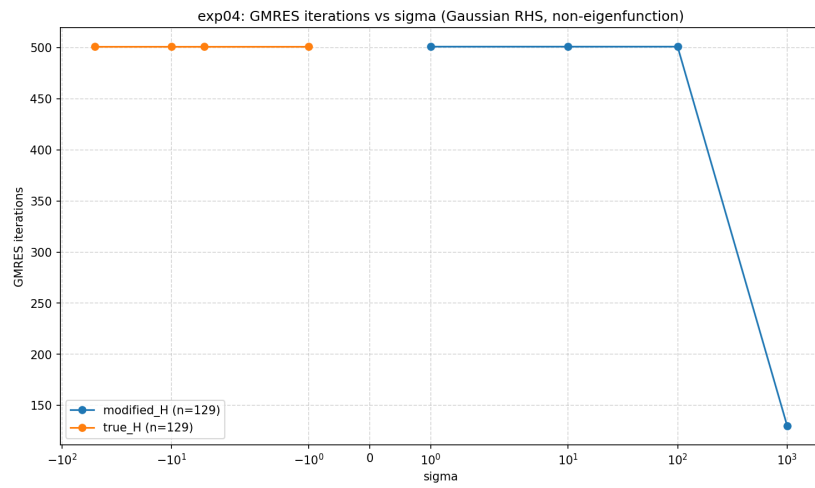
图 5: Gaussian RHS 下无预处理 GMRES 迭代次数对比
