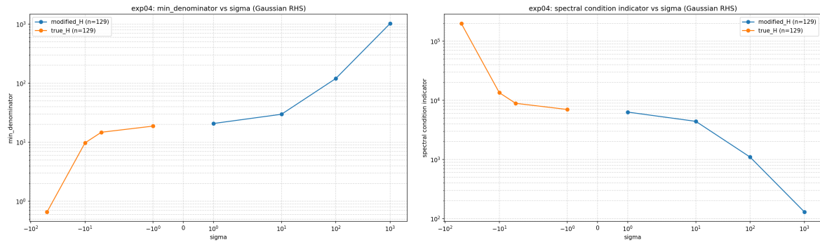
图 4: Modified/true Helmholtz 的最小频域分母与谱条件数指标
