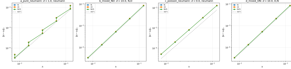
图 3: Neumann 与混合边界条件下的收敛验证
